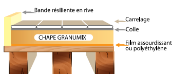
Chape sur plancher bois
