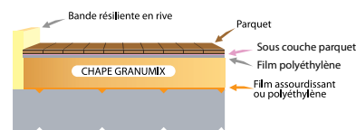
Chape sur plancher béton
